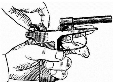
Рис. 12. Отделение боевой пружины от рамки
