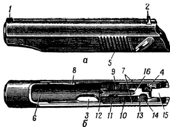
Рис. 26. Затвор:
