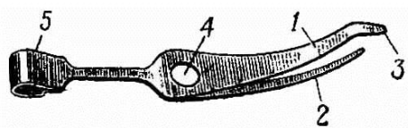
Рис. 36. Боевая пружина: 1 - широкое перо; 2 - узкое перо; 3 - отбойный конец; 4 - отверстие; 5 - защелка
