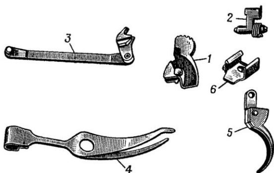
Рис. 31. Части ударно-спускового механизма:
