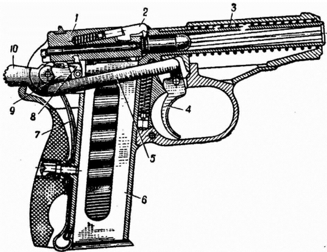
Рис. 46. Положение частей и механизмов пистолета перед выстрелом.
