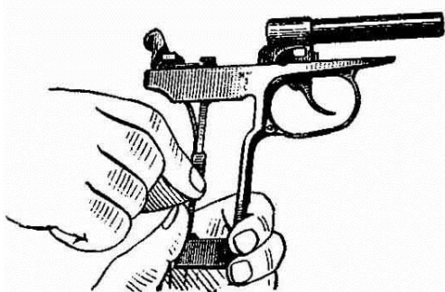
Рис. 23. Закрепление боевой пружины задвижкой
